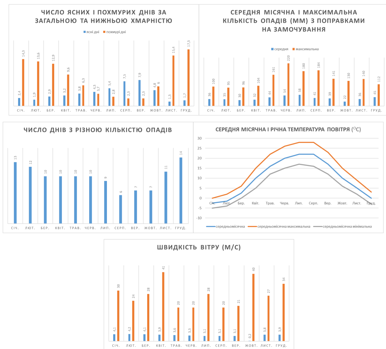
Рисунок 2.2 – Метеорологічні характеристики
