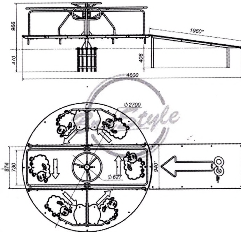
Креслення 2. Карусель для дітей з особливими фізичними можливостями ОФМ ТОВ Мірос DIO-391
