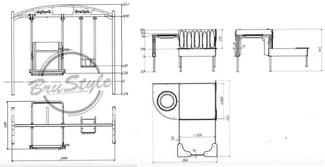
Креслення 3. Дитячий ігровий комплекс ПК2-І для людей з ОФМ
